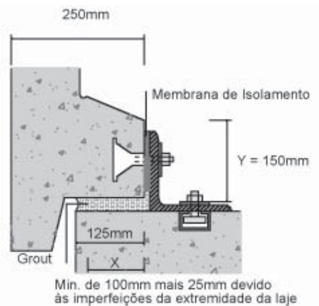
Figura 13 - Fixação da base horizontal utilizando cantoneiras (a partir de BROOKES, 1998).
