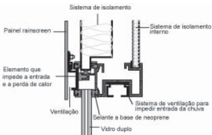
Figura 40 - Detalhe típico de fixação de painéis com rainscreen (a partir de BROOKES, 1998).
