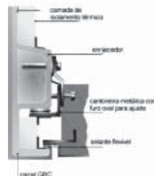
Figura 18 - Painel GRC com enrijecimento incorporado (SILVA, 1998 b ).
