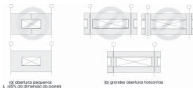
Figura 23 - Dimensões e aberturas em relação à modulação dos painéis em GRC (SILVA, 1998b).
