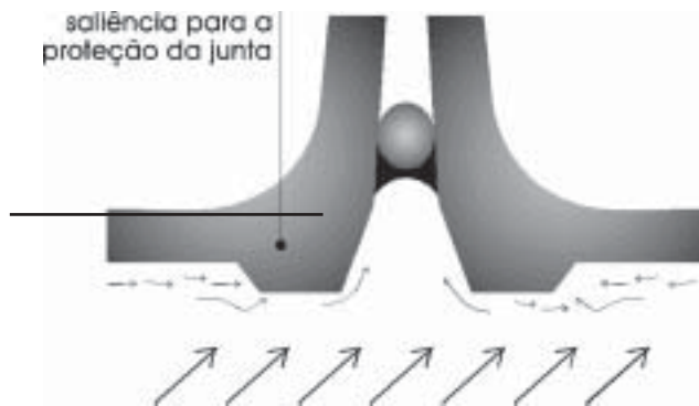
Figura 26 - Saliência na borda do painel para interceptar o fluxo da água da chuva (SILVA, 1998 b ).
