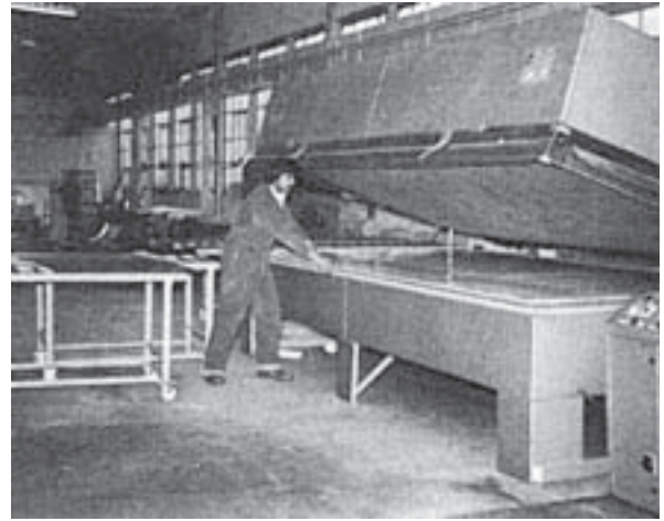
Foto 44 - Produção de painéis utilizando processo de pressão a vácuo (BROOKES, 1998).
