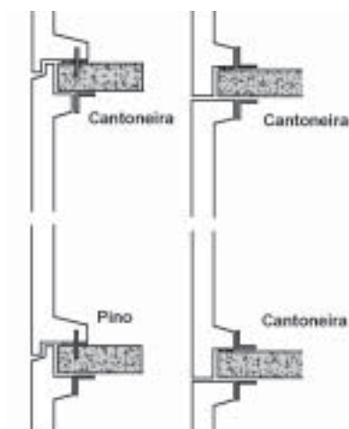
Figura 6 - Fixação de painéis de concreto.
