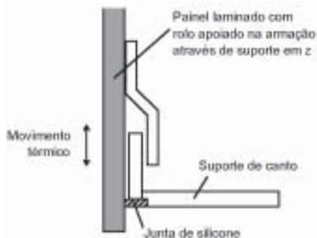
Figura 36 - Suporte dos painéis com suporte em Z
