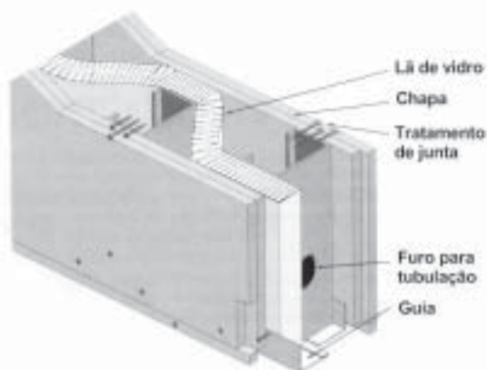
Figura 42 - Exemplo de vedação em chapas de gesso acartonado (MITIDIERI FILHO, 1997).
