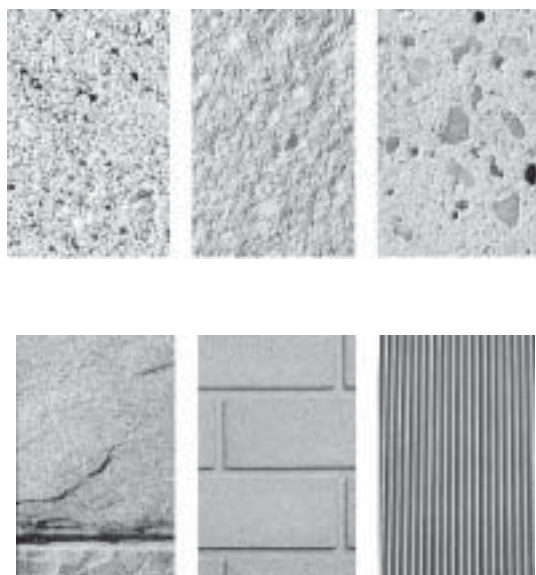
Foto 30 - Acabamentos superficiais para painéis de GRC (PCI, 1995).
