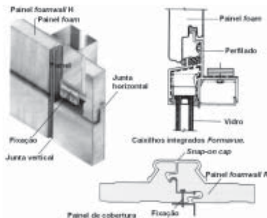
Figura 32 - Painéis metálicos compósitos (FINESTRA 1997 2 ).
