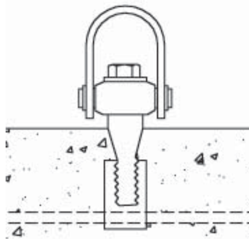
Figura 4 - Insert de içamento em forma de elo
