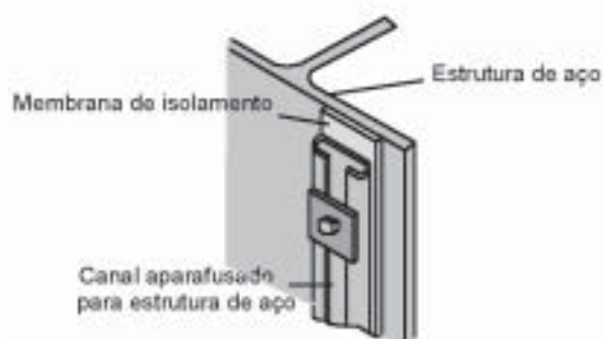
Figura 8 - Isolamento físico (vertical) entre metais não similares (DAWSON, 1995).
