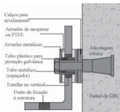
Figura 27 - Fixação no GRC com conector com entalhe e ancoragem cônica (CIRIA, 1992 a , BROOKES, 1998).
