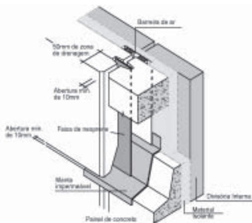
Figura 1 - Detalhe de junta aberta e drenada com faixa vertical de neoprene ( baffle strip ).
