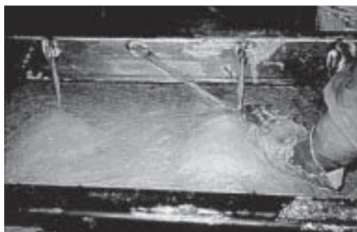
Foto 29 - Incorporação do enrijecimento metálico a painéis GRC (PCI, 1995).
