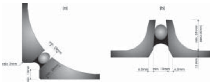
Figura 24 - Detalhes típicos de juntas entre painéis: (a) junta de canto do painel; (b) junta entre painéis (a partir de PCI, 1994).
