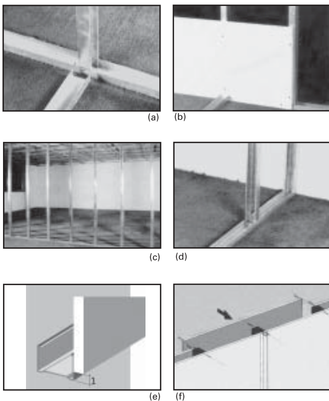
Foto 44 - Seqüência de montagem: a e b colocação das guias, c e d colocação dos montantes, e folga entre chapas e piso (MITIDIERI FILHO, 1997) e f detalhe dos desencontros das juntas (MITIDIERI FILHO, 1997).
