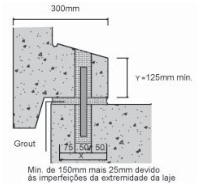
Figura 12 - Fixação da base horizontal utilizando pinos (a partir de BROOKES, 1998).
