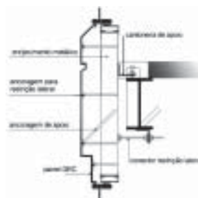
Figura 19 - Painel GRC enrijecido por uma estrutura metálica leve (stud frame) (SILVA, 1998 b ).
